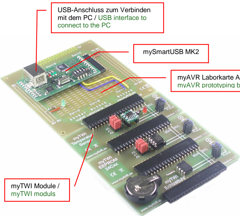
Abbildung / picture: mySmartUSB MK2 mit TWI-Modulen / mySmartUSB MK2 with TWI-moduls
