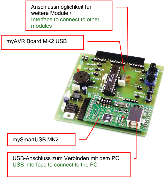
Abbildung / picture: mySmartUSB mit myAVR-Board MK2 USB / mySmartUSB with myAVR-Board MK2 USB
